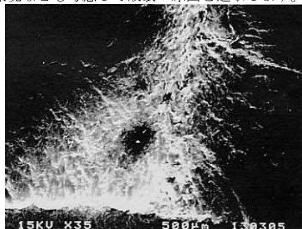
延性破壊
