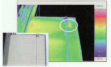
モルタル外壁の浮き
