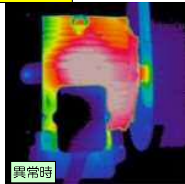
ポンプモーターの異常
