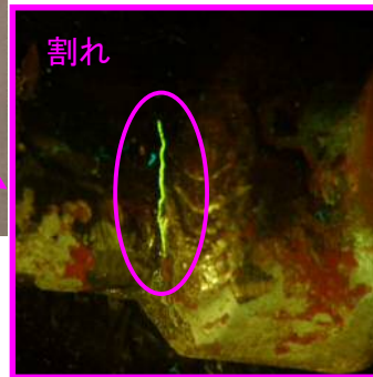
磁粉探傷試験状況
