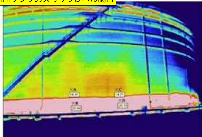
石油タンクのスラッジレベル調査
