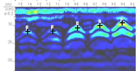
+印は鉄筋からの反射像
