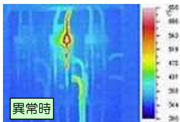
電源切替板の不良
