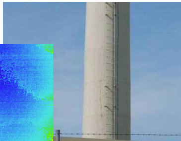
煙突の診断
