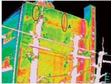
モルタル外壁の浮き
