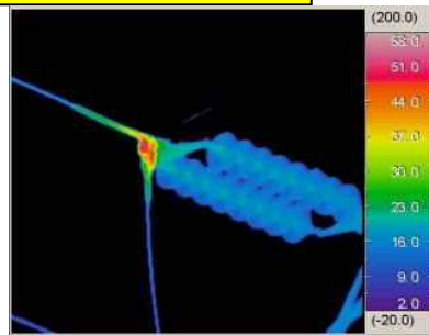
送電線(直線リ-フ)の不良
