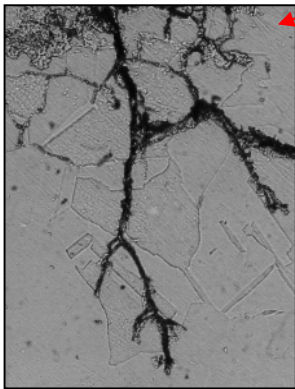
粒内貫通
